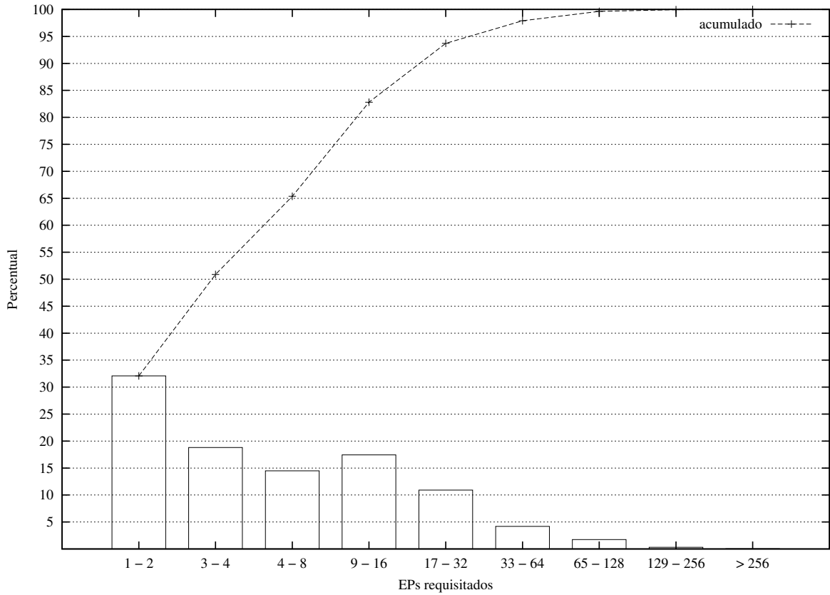
Figura 4.6: Histograma da quantidade de EPs requisitados (SDSC95)
