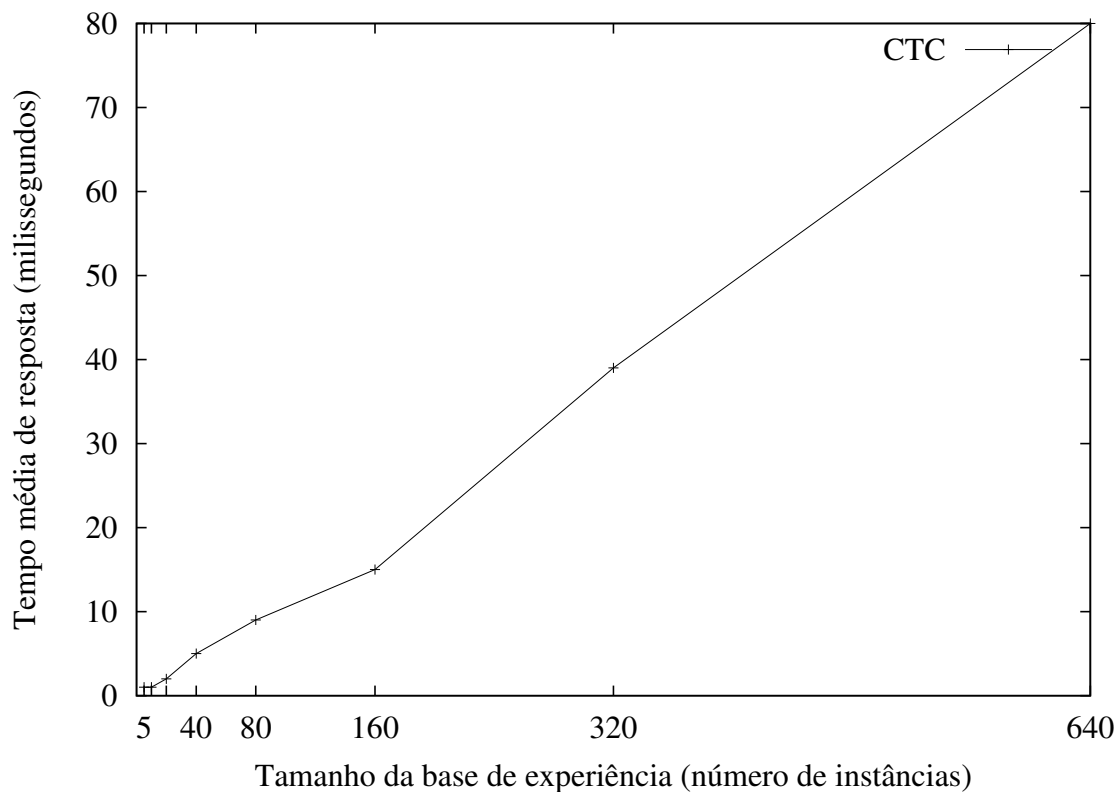
Figura 6.2: Tempo de resposta do algoritmo IBL
