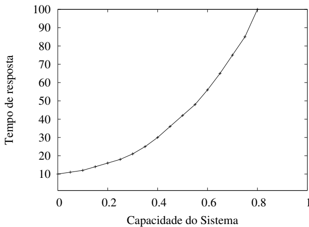
Figura 2.2: Tempo de resposta em relação à utilização do sistema
