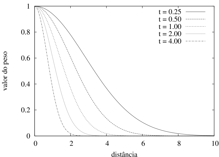
Figura 3.5: Função gaussiana com 4 valores diferentes de t
