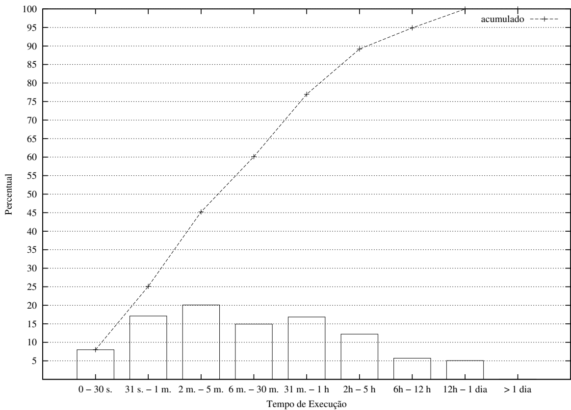
Figura 4.3: Histograma do tempo de execução das aplicações (SDSC2000)
