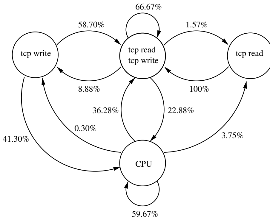
Figura 5.6: Diagrama de estados para a aplicação SP (tamanho de problema B )
