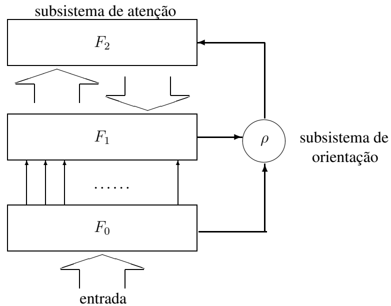
Figura 3.3: Arquitetura básica das redes ART
