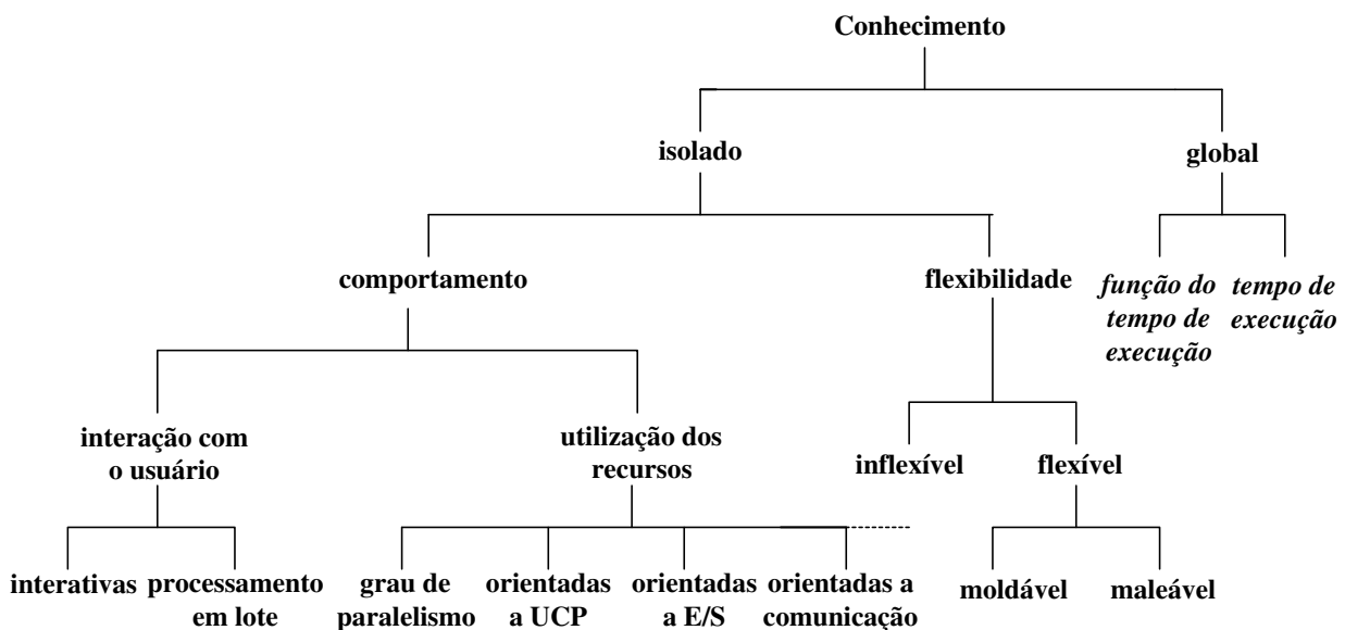
Figura 2.5: Classificação do conhecimento sobre as aplicações paralelas
