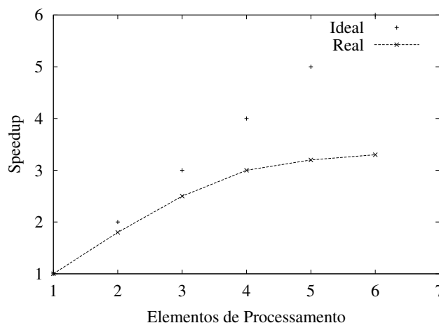
Figura 2.1: Speedup de uma aplicação paralela
