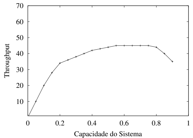
Figura 2.3: Throughput em relação à utilização do sistema
