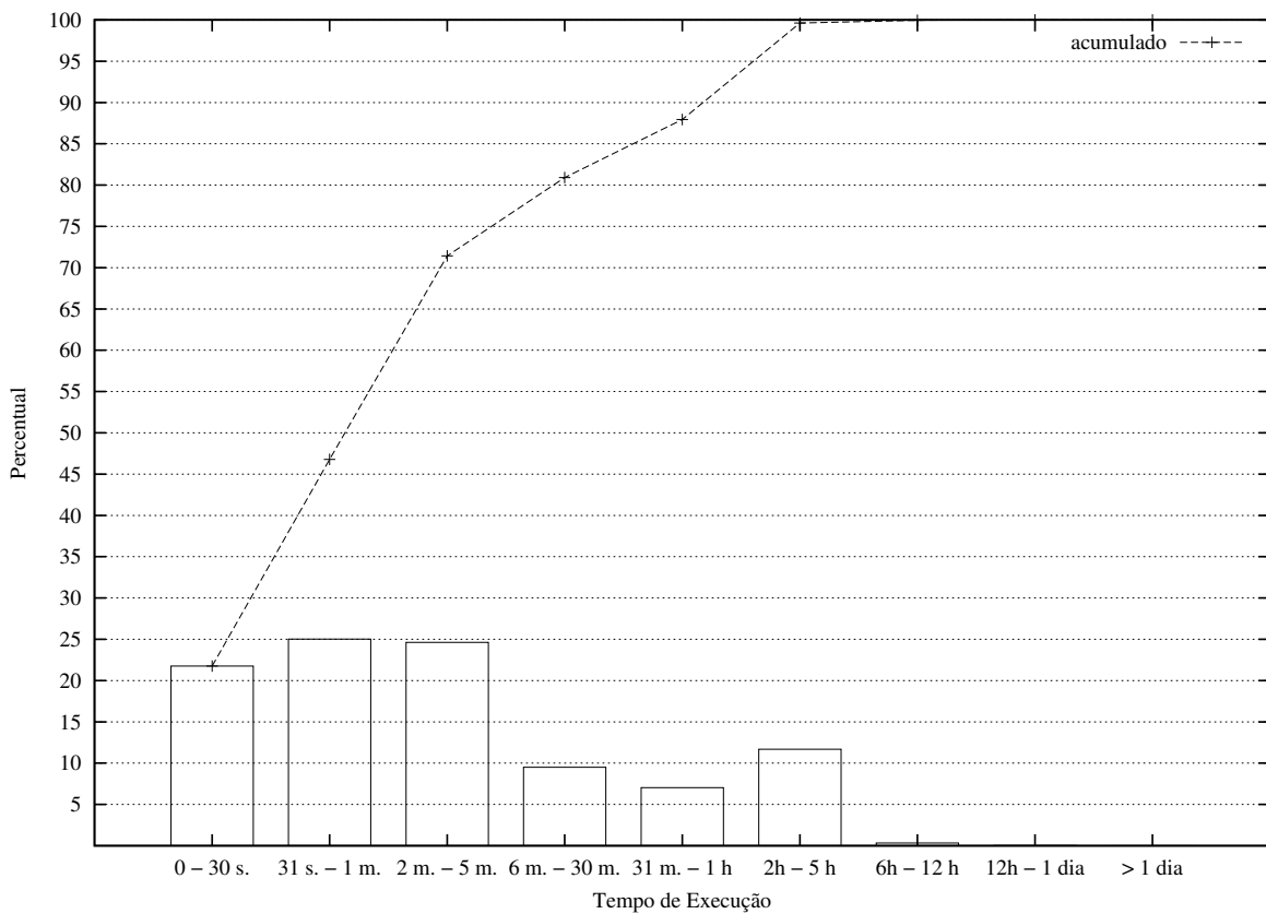
Figura 4.5: Histograma do tempo de execução das aplicações (LANL)
