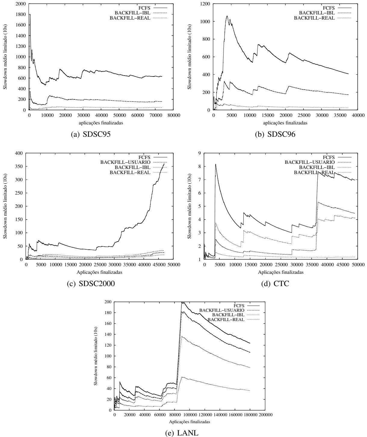
Figura 7.1: Desempenho dos algoritmos de escalonamento avaliados
